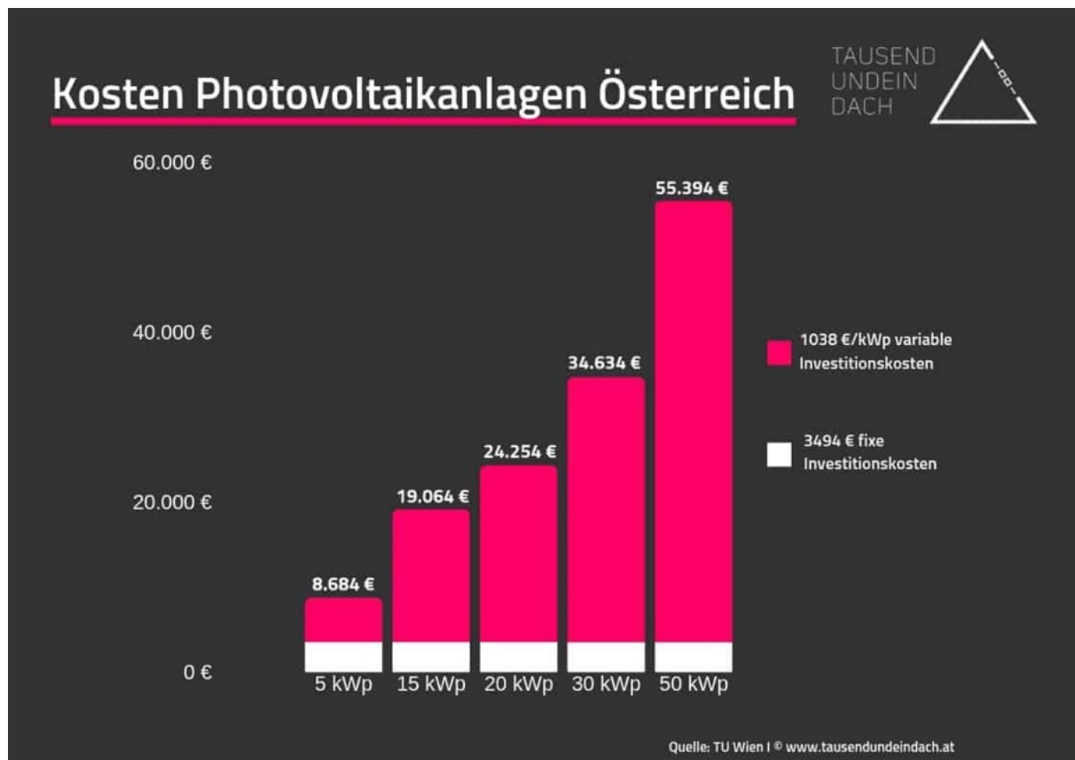
Abbildung 8: Kosten für Photovoltaikanlagen in Österreich (Dachgold, 2020a)
